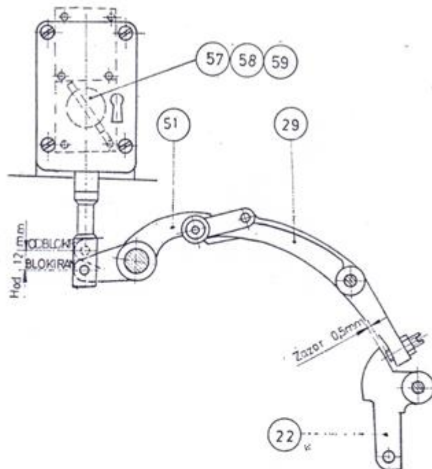
Slika 4. Blokada uključnja »BOURE« ili »KASTELL« bravom BNR-1B-1M (100208)
