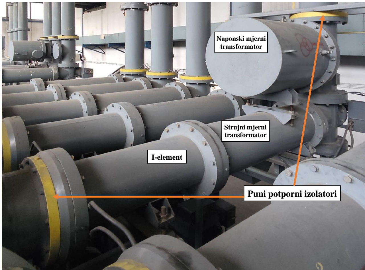
Slika 5. Polje DV 110 kV Pale - Gasna zona 2 sa induktivnim naponskim transformatorom u fazi 4
